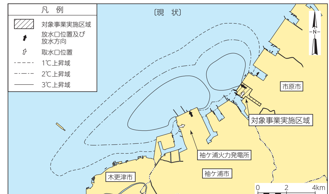
温排水拡散予測結果（海表面）
