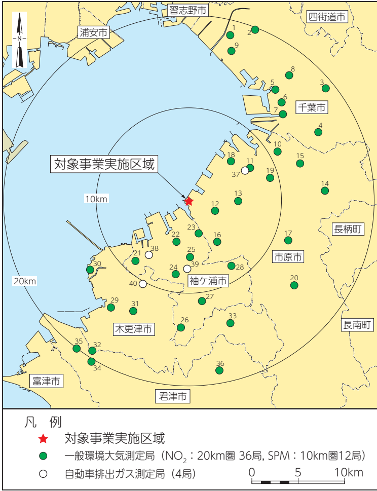
大気質測定局の位置
